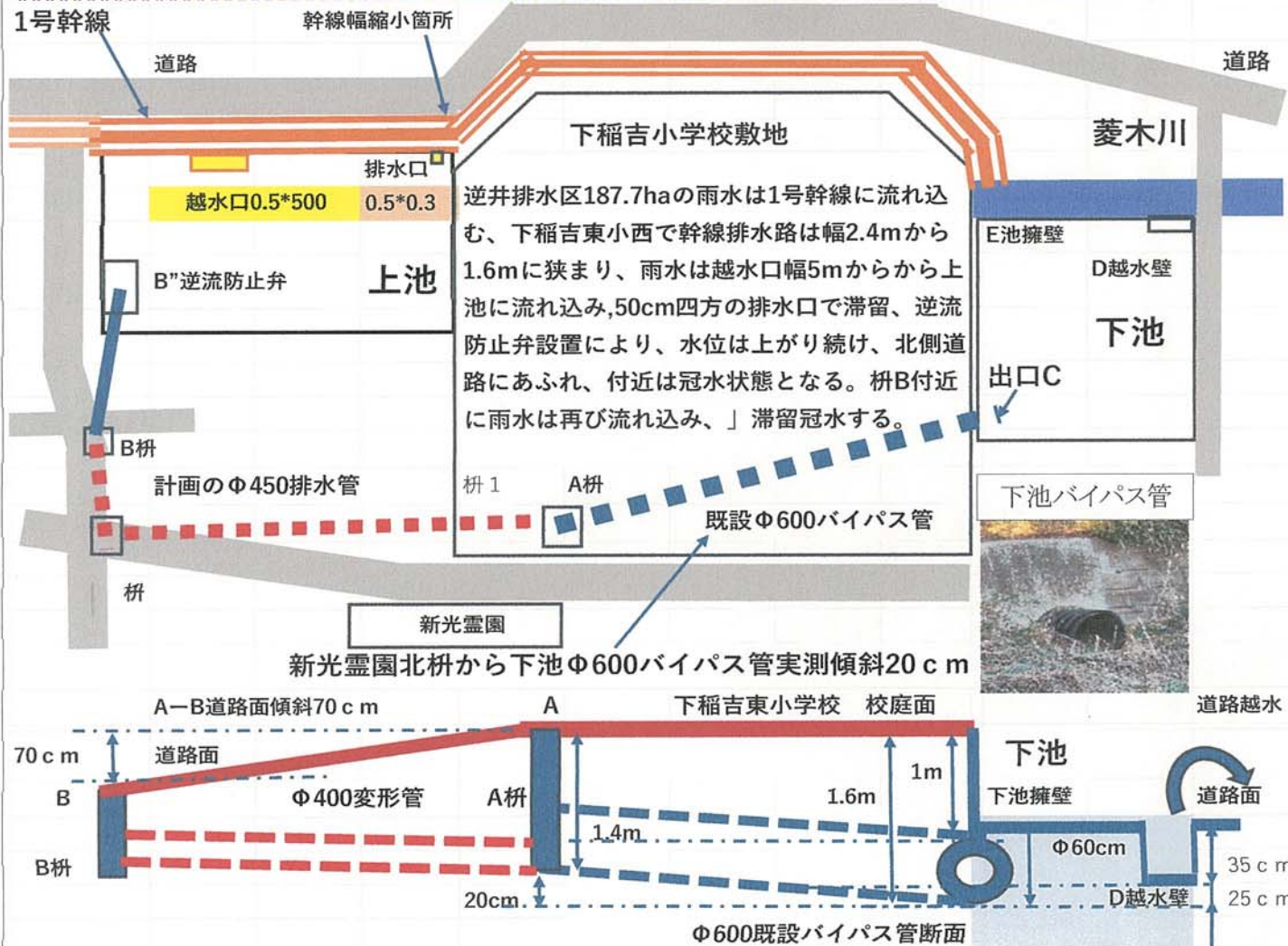
パイパス管下端から25cmの高さに越水壁上面がある。下池擁壁まで水位が上がると管出口は水没する。
